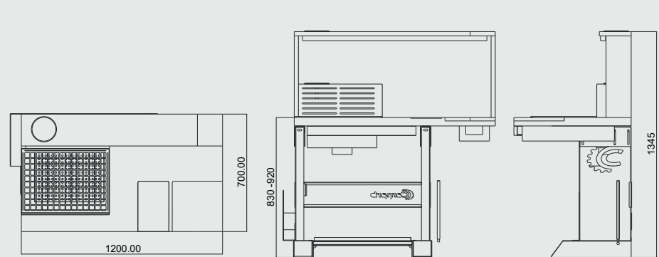
Connessione superiore per l'aspirazione centralizzata / Upper connection for centralized suction
